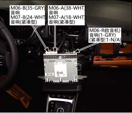
53.仪表板中央
