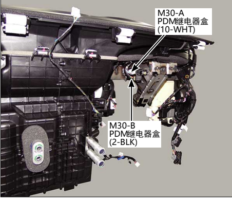
65.仪表板后左
