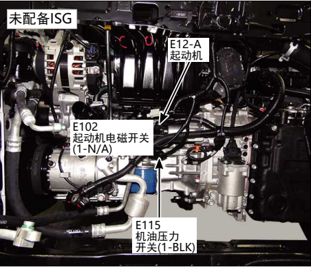
26.发动机左侧
