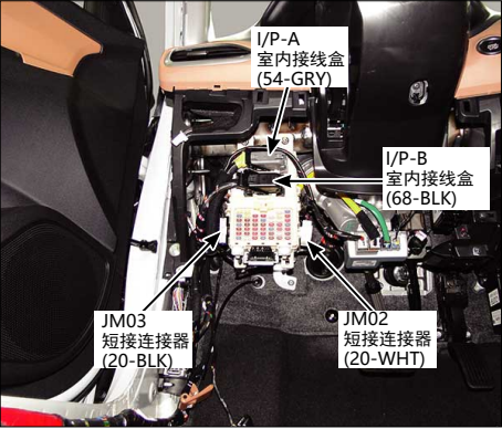
41.仪表板左侧
