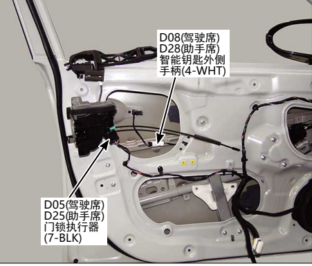
107.前车门
