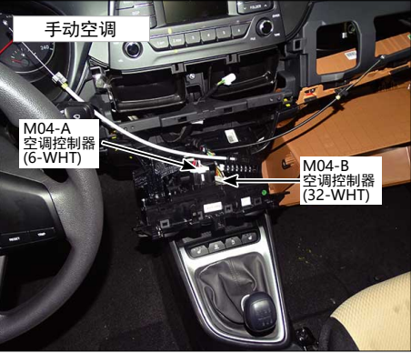
54.仪表板中央
