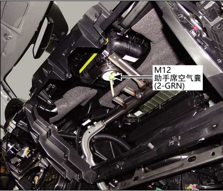
61.仪表板右侧
