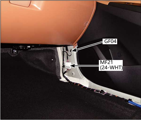
63.仪表板右侧
