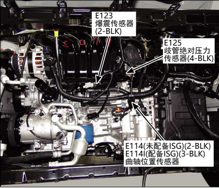
28.发动机左侧
