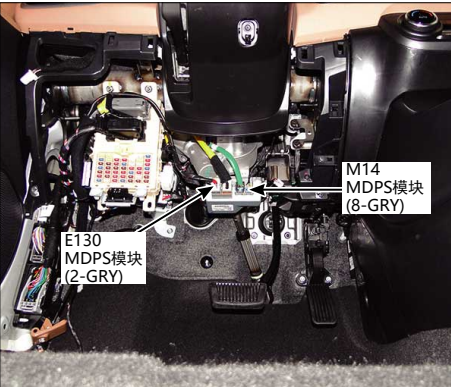
48.转向柱
