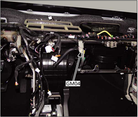
57.仪表板中央
