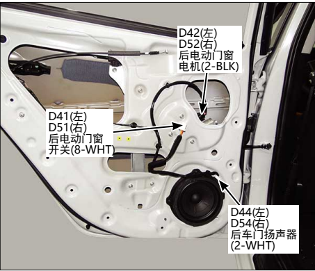
110.后车门
