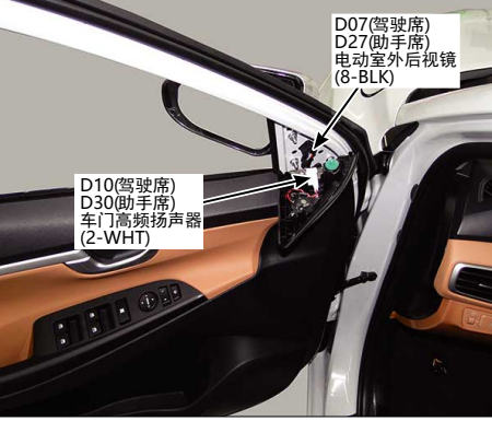
106.前车门
