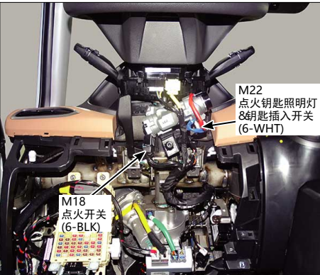
45.转向柱
