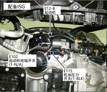
27.发动机左侧
