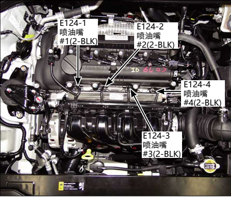
23.发动机顶部
