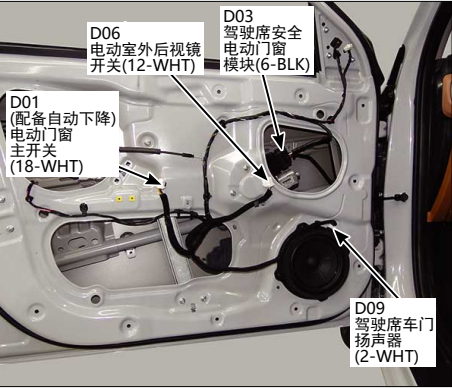
105.驾驶席车门
