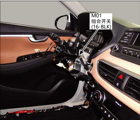
47.转向柱
