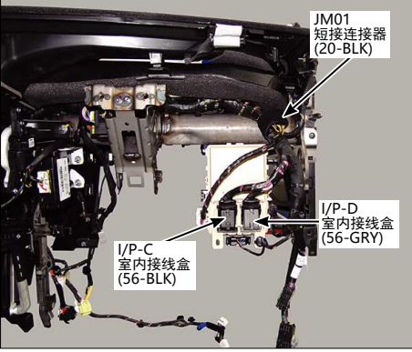
64.仪表板后左
