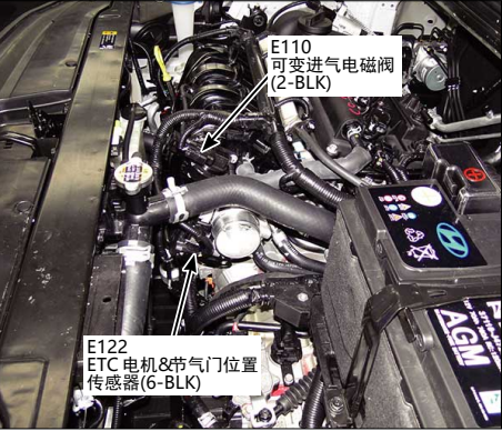
29.发动机后左
