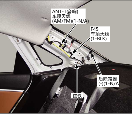
90.后右立柱
