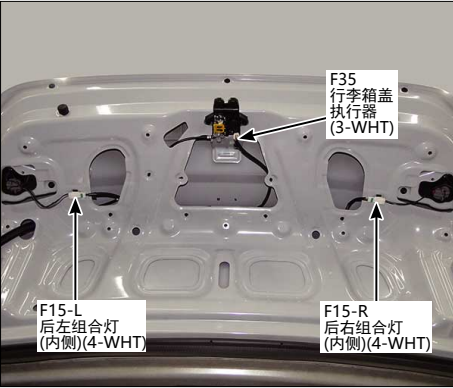
97.行李箱盖
