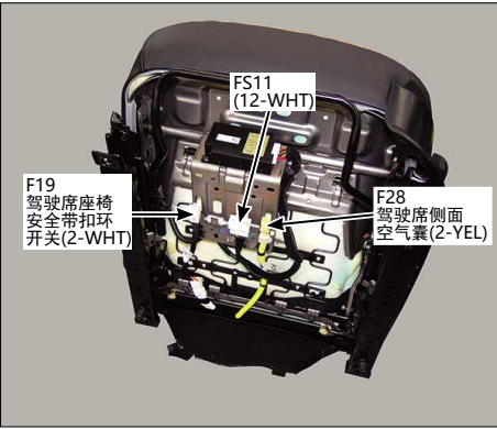
82.驾驶席座椅
