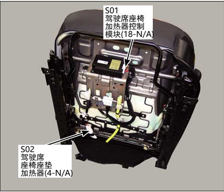
83.驾驶席座椅
