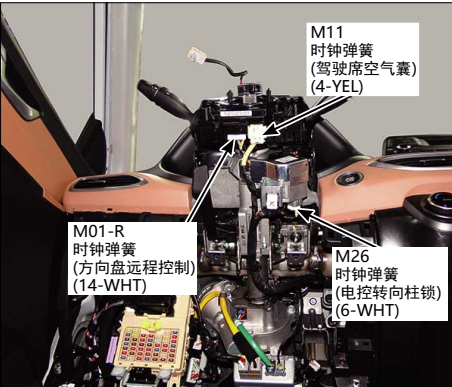
46.转向柱
