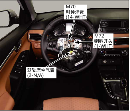
42.方向盘
