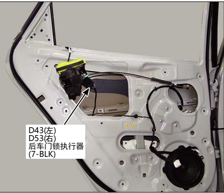
111.后车门
