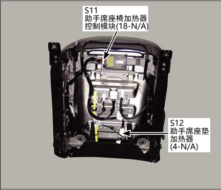
85.助手席座椅
