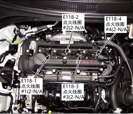
24.发动机顶部
