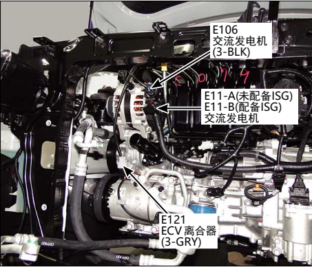
25.发动机前左
