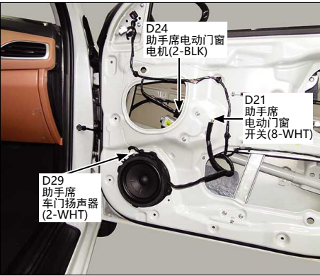
109.助手席车门
